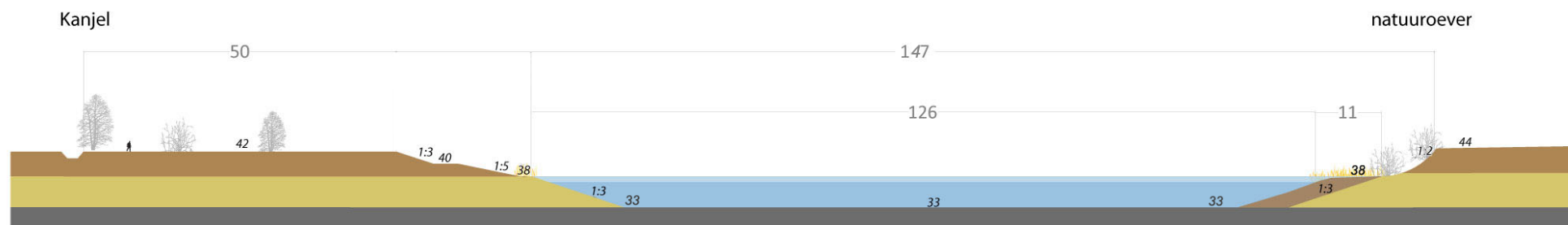
Profiel A - A'
