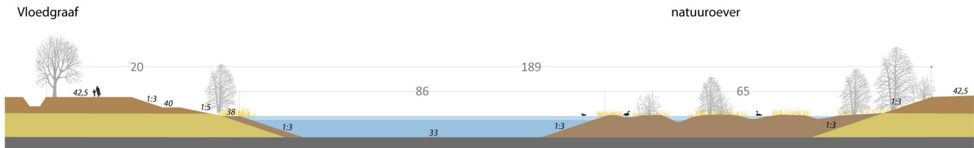
Profiel B - B'
